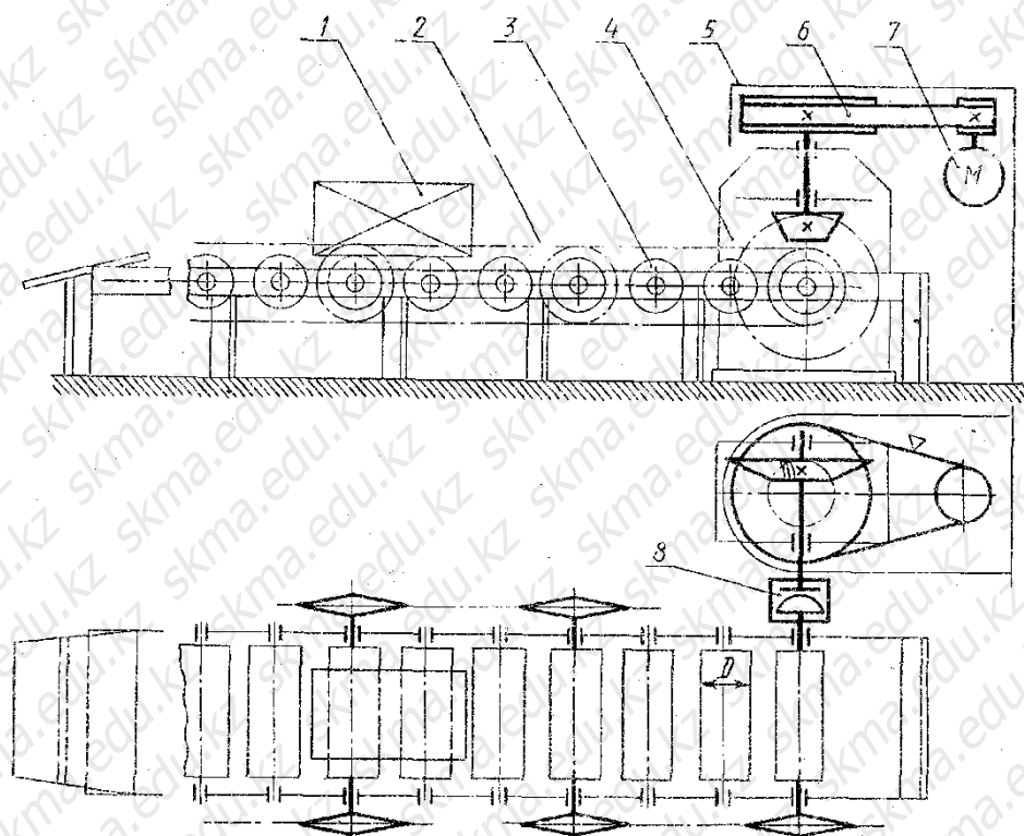
1—груз; 2—приводная цепь; 3—ролик; 4—конический редуктор; 5—ограждение; 6—клиноременная передача; 7—двигатель; 8—цепная муфта
