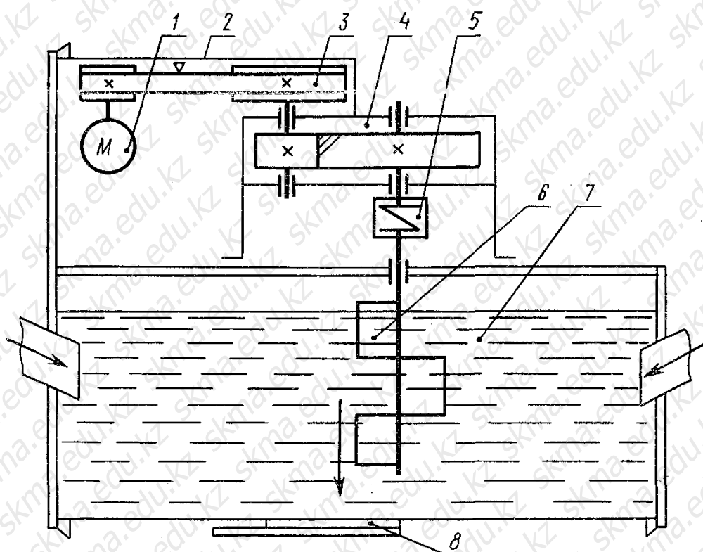
1—двигатель; 2—ограждение; 3—клиноременная передача; 4—цилиндрический редуктор; 5—упругая муфта с торообразной оболочкой; 6—мешалка; 7—смесь; 8—задвижка
