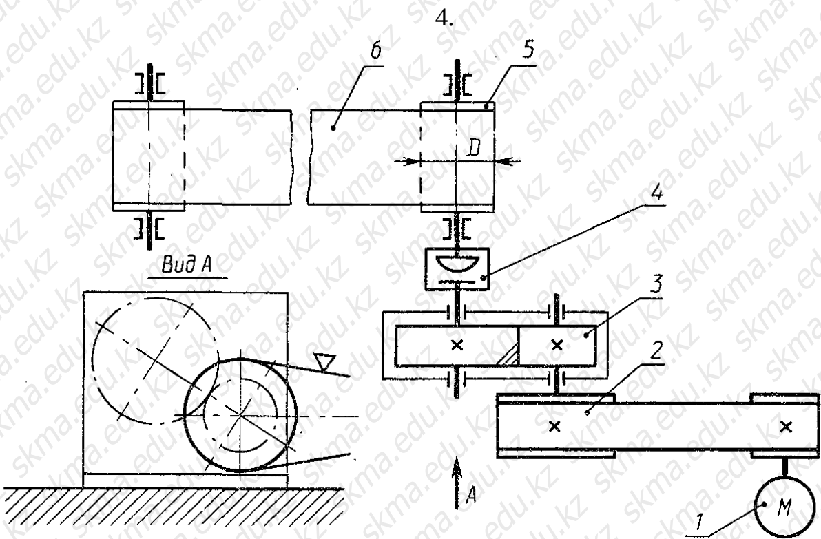
1 — двигатель; 2 — клиноременная передача; 3 — цилиндрический редуктор; 4 — цепная муфта; 5 — барабан; 6 — ленты конвейера
